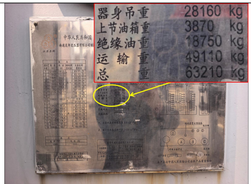
2 号主变铭牌
