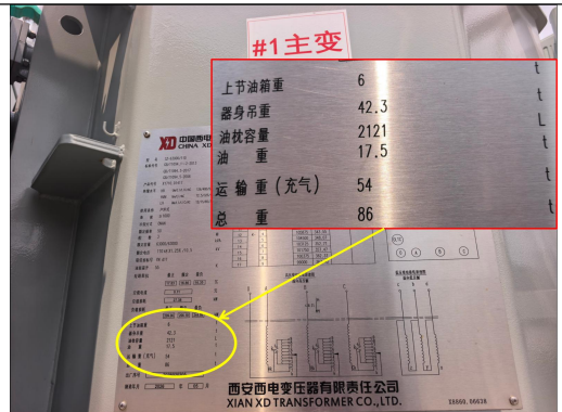
1 号主变铭牌
