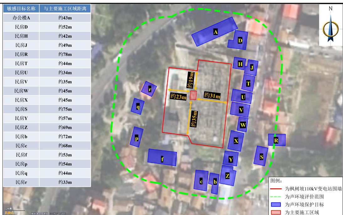
图 4-2 枫树坡 110kV 变电站施工区域及环境保护目标分布图
