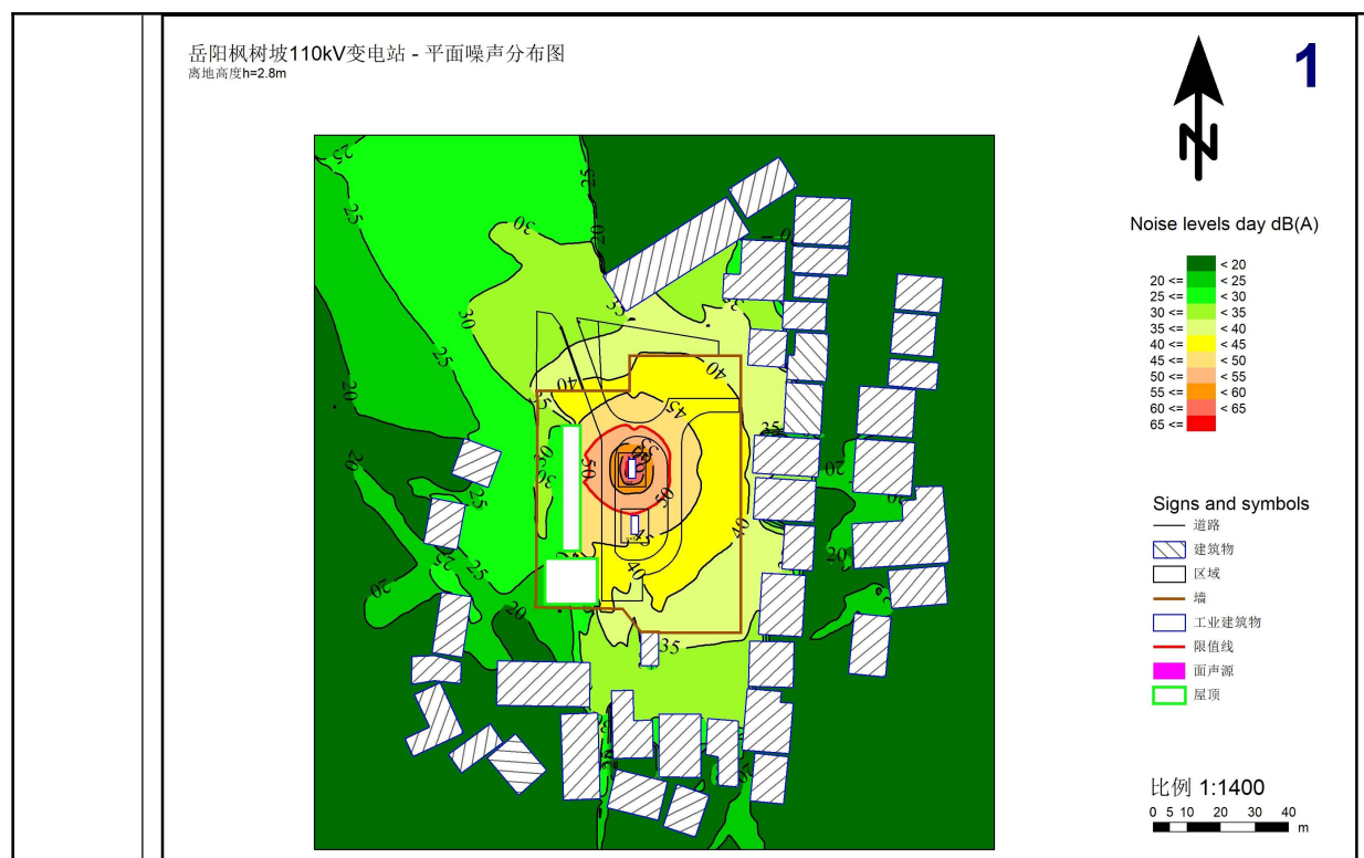
图 4-5 枫树坡变电站本期规模噪声贡献值等值线图（围墙上方 0.5m）
