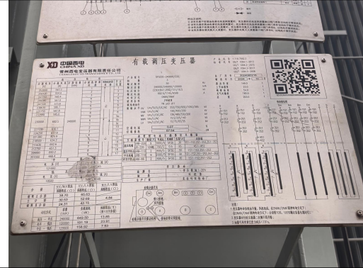
2 号主变铭牌
