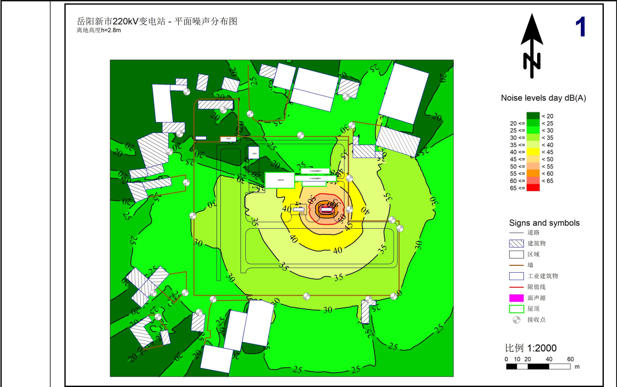
图 4-5 新市变电站本期规模噪声贡献值等值线图（围墙上方 0.5m）
