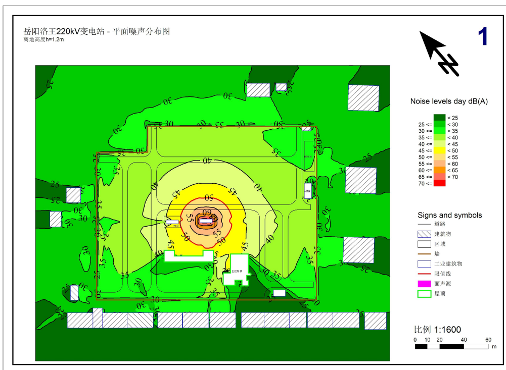
图 4-5 洛王变电站本期规模噪声贡献值预测等值线图（地面上方 1.2m）
