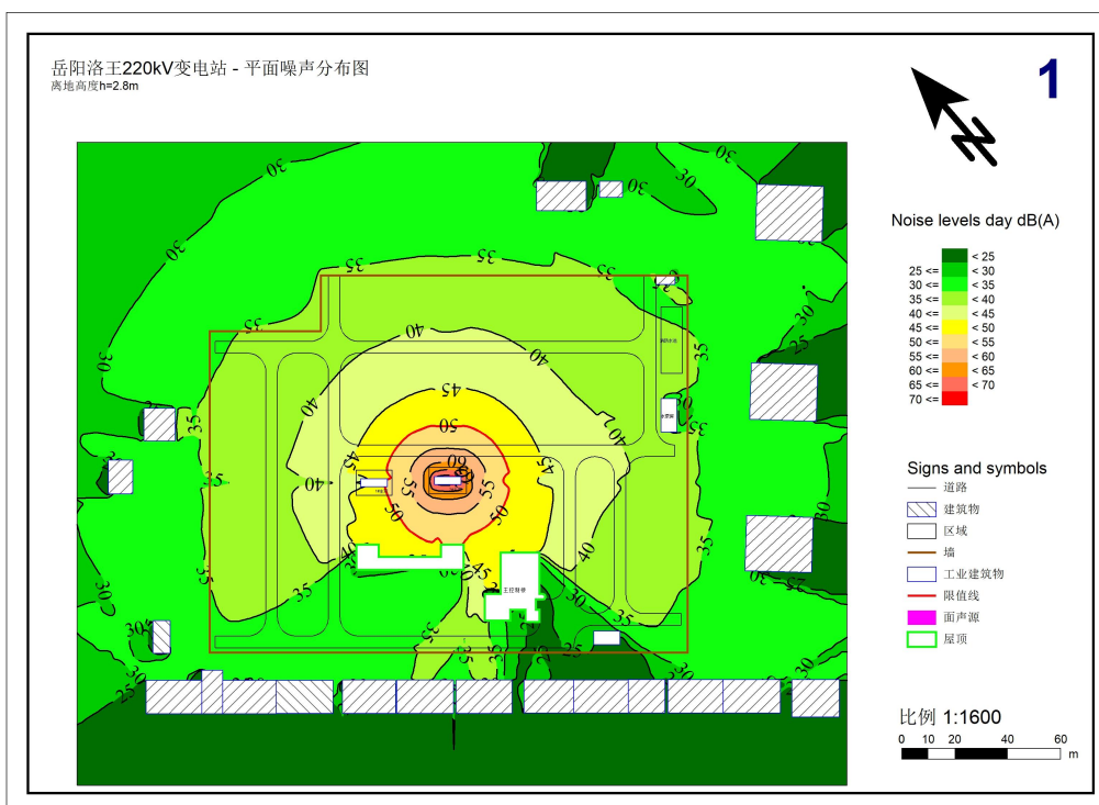
图 4-6 洛王变电站本期规模噪声贡献值预测等值线图（围墙上方 0.5m）
