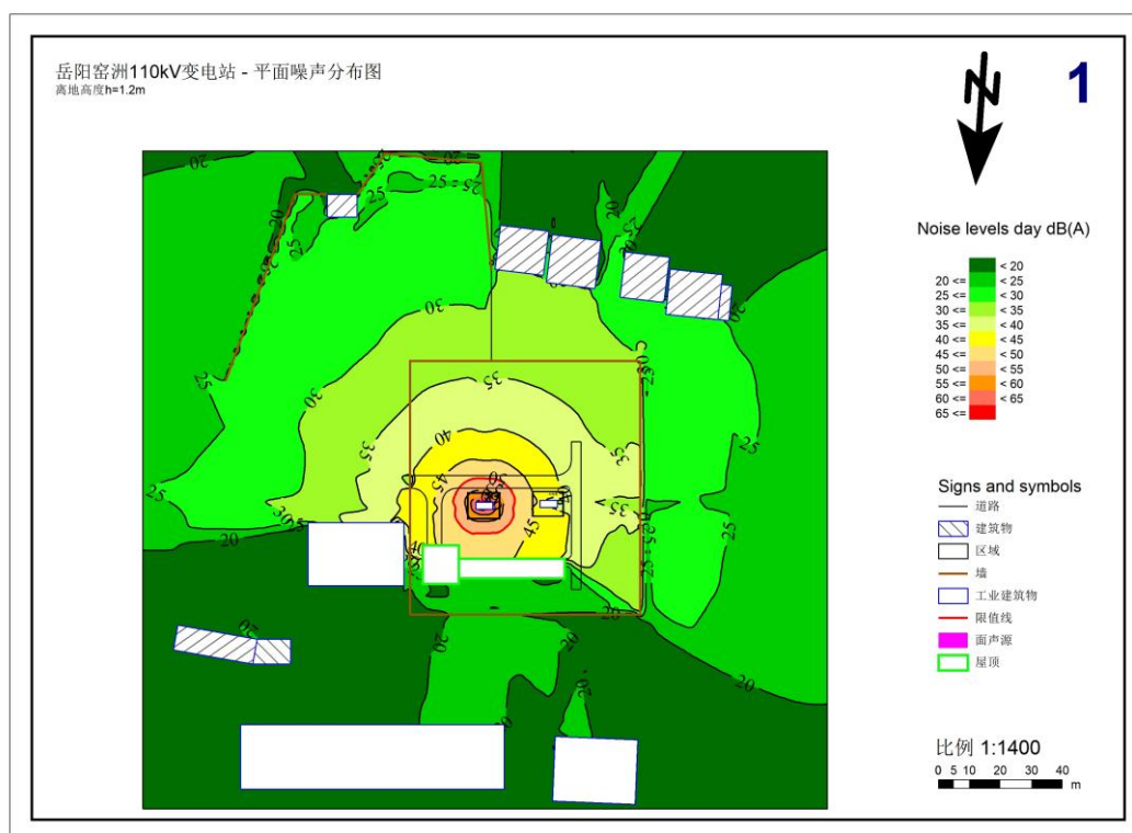
图 4-5 窑洲变电站本期规模噪声预测等值线图（地面上方 1.2m）
