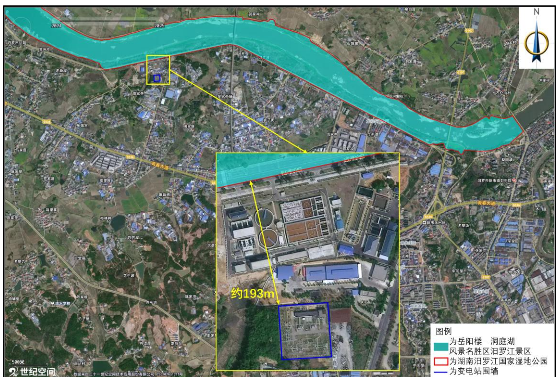
图 3-5 本工程与岳阳楼—洞庭湖风景名胜区、湖南汨罗江国家湿地公园相对位置关系图
