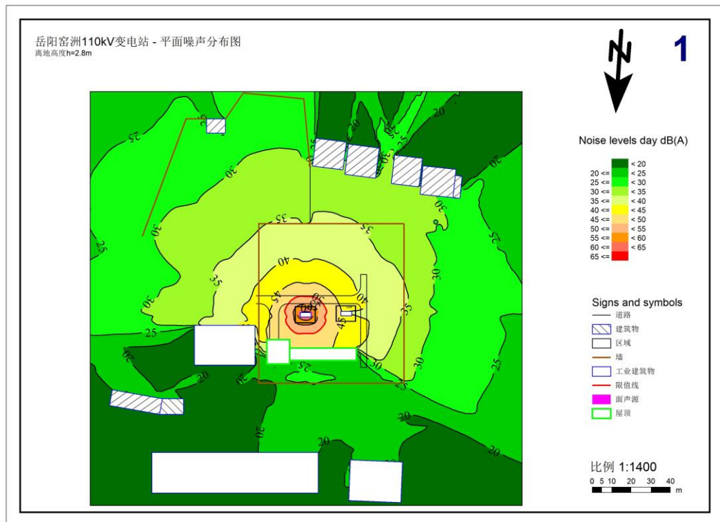
图 4-6 窑洲变电站本期规模噪声预测等值线图（围墙上方 0.5m）
