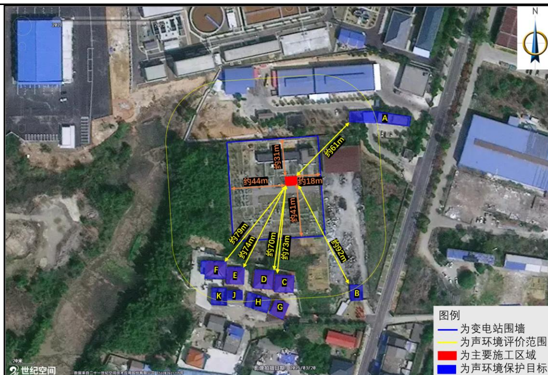
图 4-2 窑洲 110kV 变电站施工区域及环境保护目标分布图
