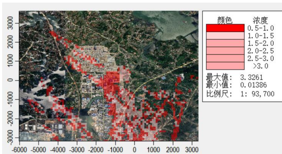
图 8.2-8 SO 2 小时值浓度贡献值预测结果分布图 (μg/m 3 )
