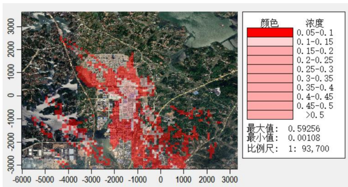
图 8.2-9 SO 2 日均值浓度贡献值预测结果分布图 (μg/m 3 )
