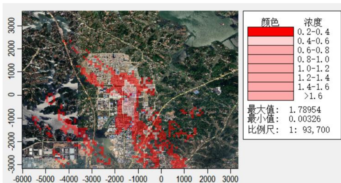
图 8.2-12 NO x 日均值浓度贡献值预测结果分布图 ( \mu\text{g}/\text{m}^3 )
