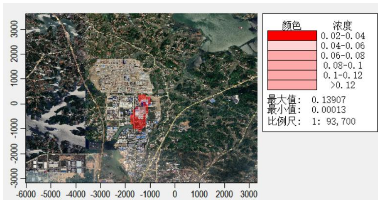
图 8.2-10 SO 2 年均值浓度贡献值预测结果分布图 (μg/m 3 )
