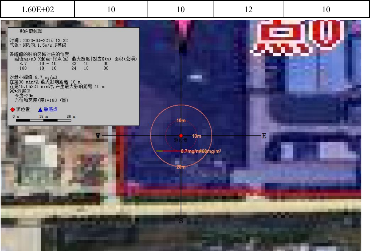
图 9.7-1 事故排放状态下硫酸雾毒性终点浓度的最大影响范围图（最不利气象条件）
