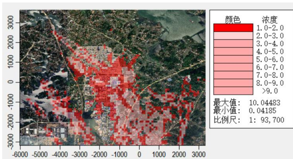
图 8.2-11 NO x 小时值浓度贡献值预测结果分布图 ( \mu\text{g}/\text{m}^3 )
