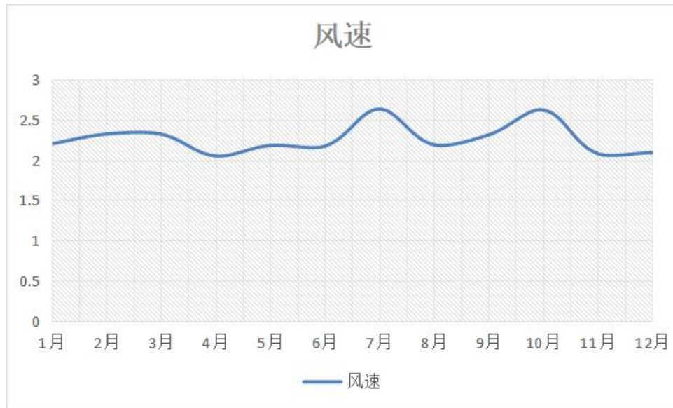
图 8.2-2 2021 年各月平均风速变化曲线图
