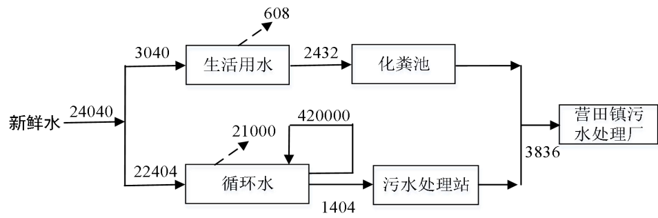
图 2-1 水平衡图 (最大用水量, 单位: m³/a)
