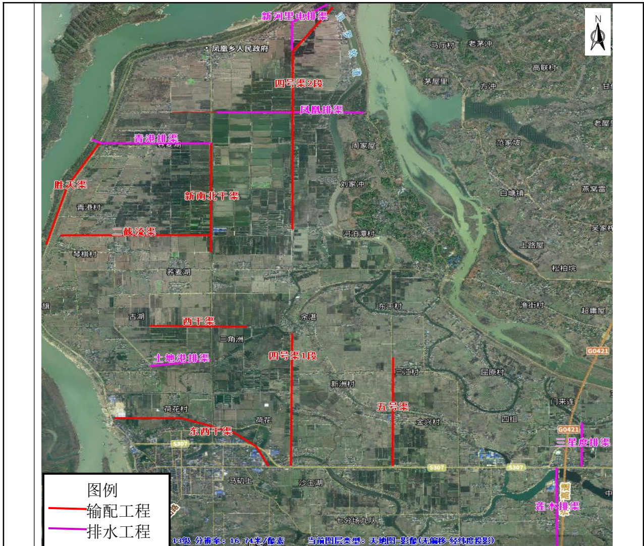
图 2-1 输配工程和排水工程总体布置图
