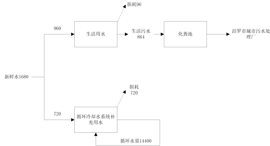
图 2.3-1 水平衡图（单位：t/a）
