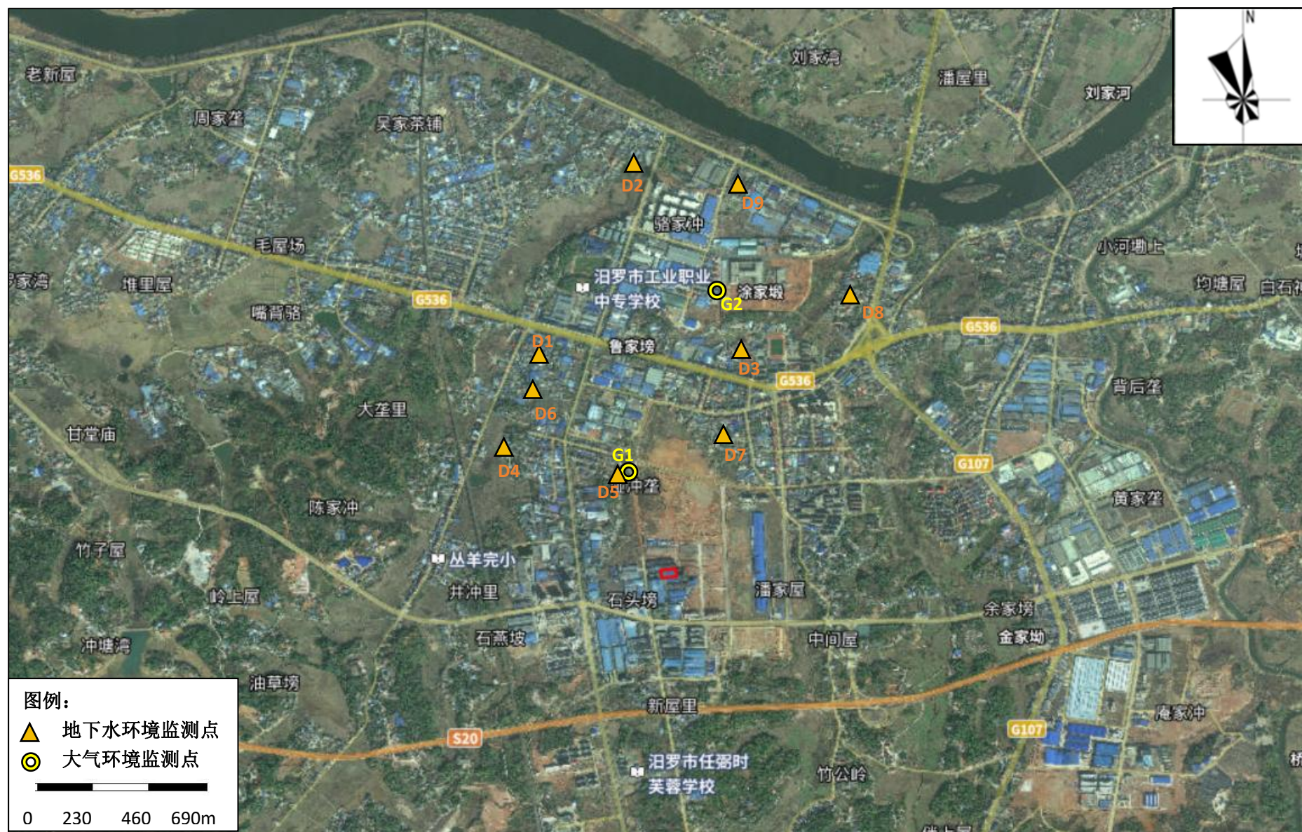
附图 2 引用大气和地下水现状监测点位图
