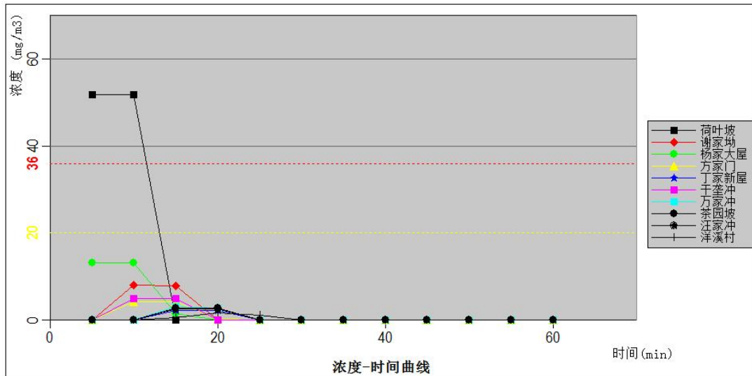
图 7.3.6-1a 主要关心点 HF 浓度随时间变化情况图（最不利气象条件）
