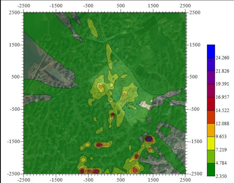
图 7.2.1.7-13a 甲醇小时值浓度叠加在建源及环境背景浓度预测结果分布图 ( \mu\text{g}/\text{m}^3 )
