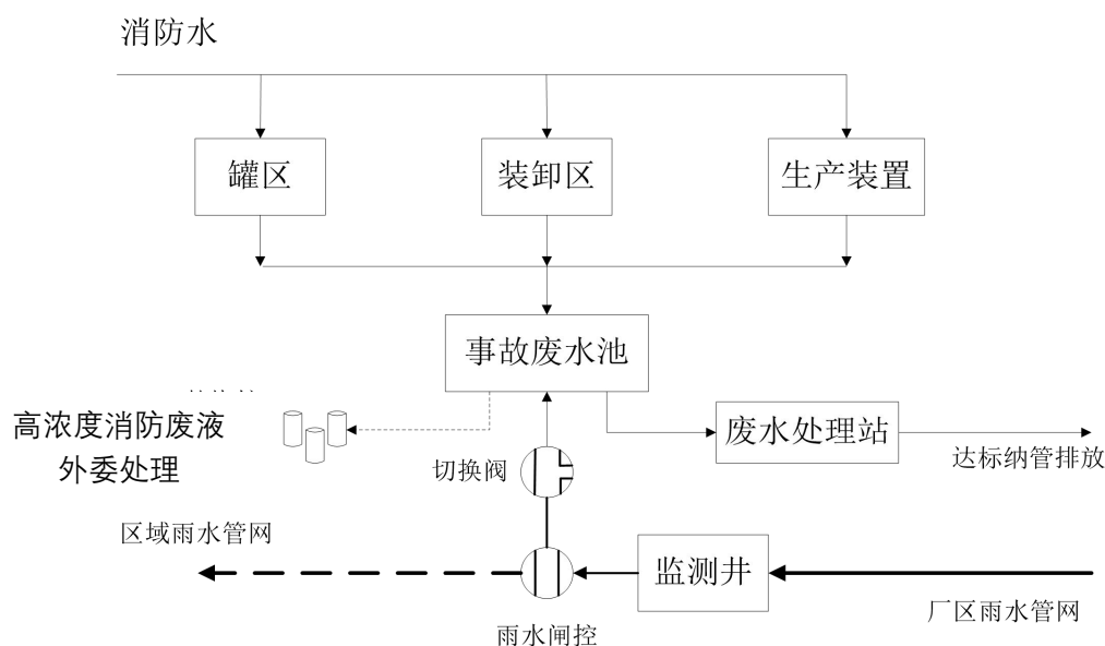
图 7.3.7-2 事故时污水收集管网示意图
