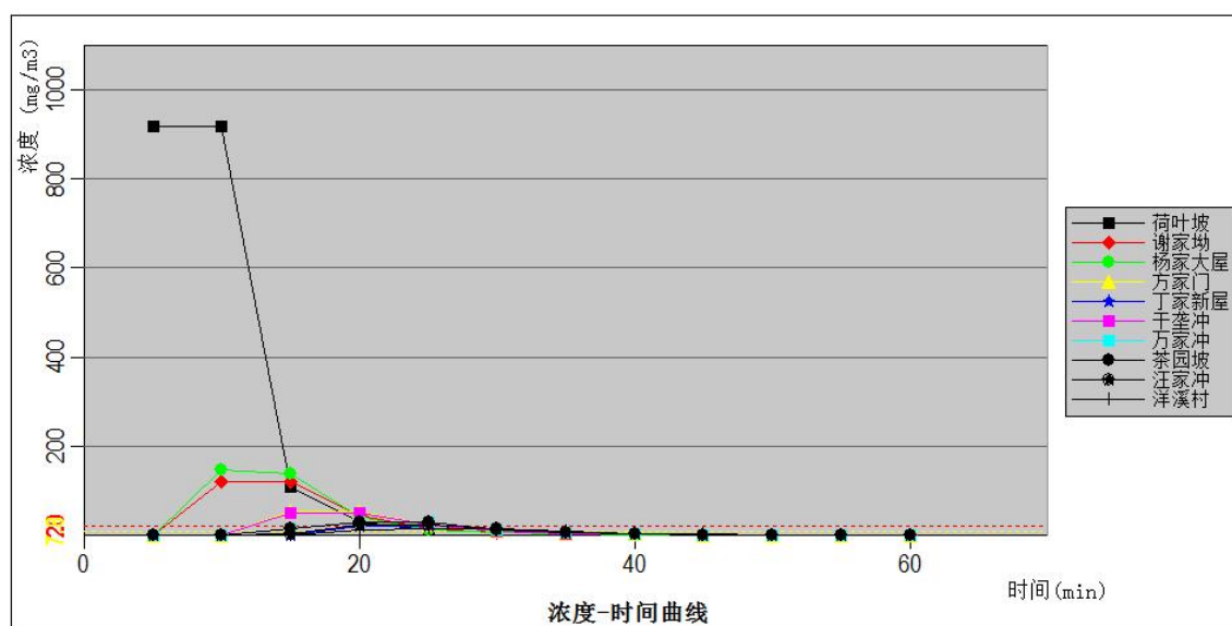
图 7.3.6-2a 主要关心点 F2 浓度随时间变化情况图（最不利气象条件）
