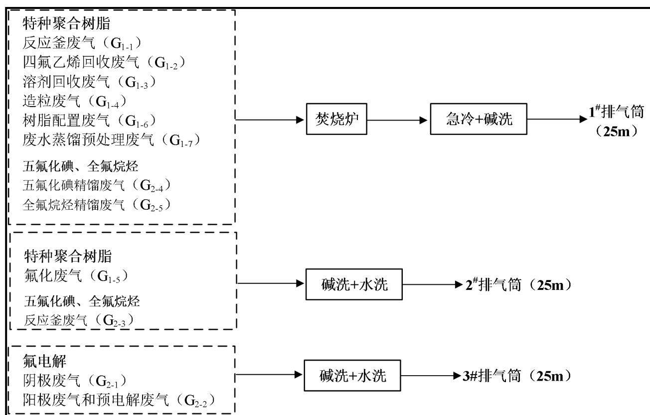
图 8.1-1 有组织废气处理措施及去向示意图
