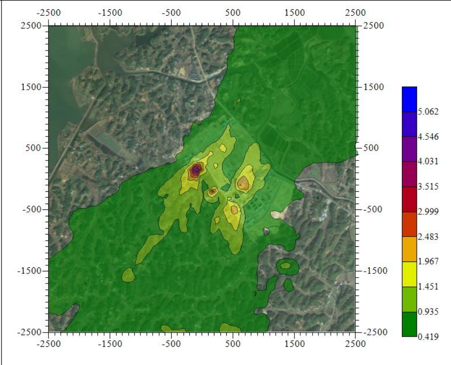
图 7.2.1.7-13b 甲醇日均值浓度叠加在建源及环境背景浓度预测结果分布图 ( \mu\text{g}/\text{m}^3 )
