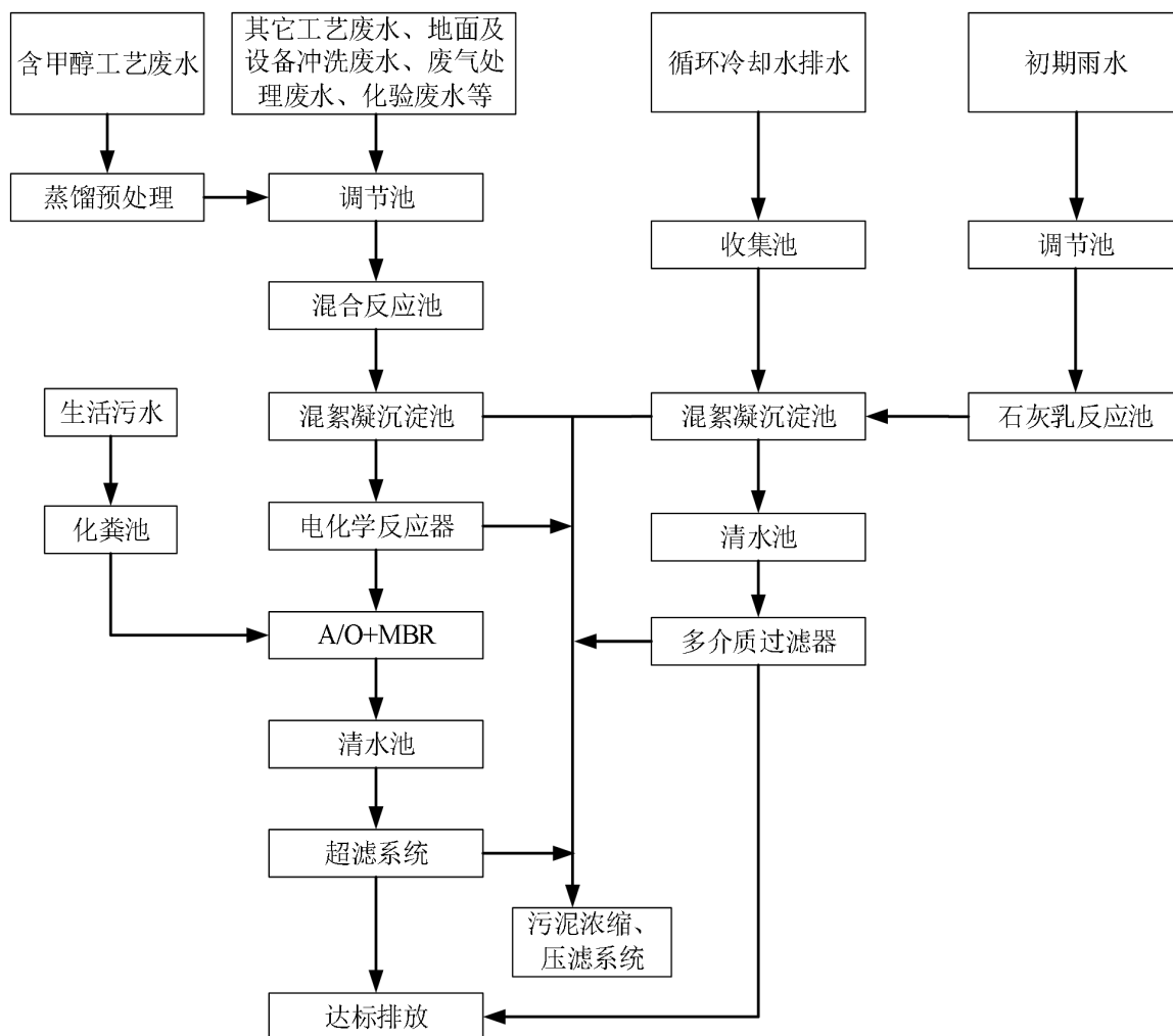
图 8.2-1 废水处理流程示意图
