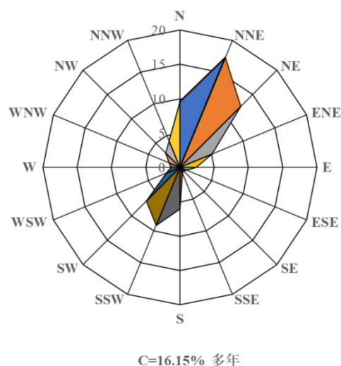
图 7.2.1.4-1 临湘气象站近 20 年风向玫瑰图 单位：%
