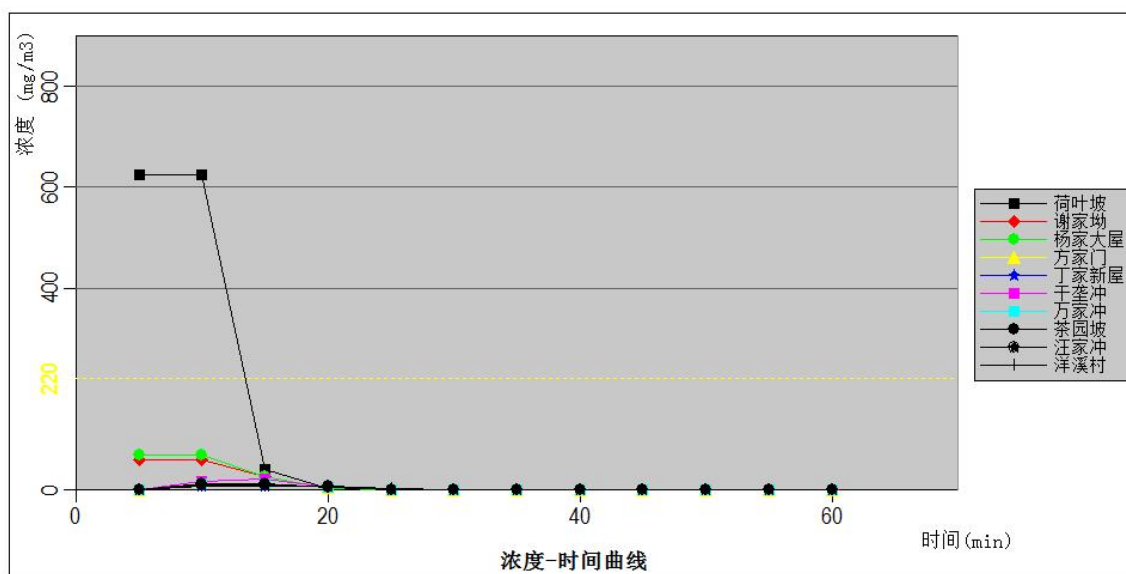
图 7.3.6-3b 主要关心点四氟乙烯浓度随时间变化情况图（最常见气象条件）
