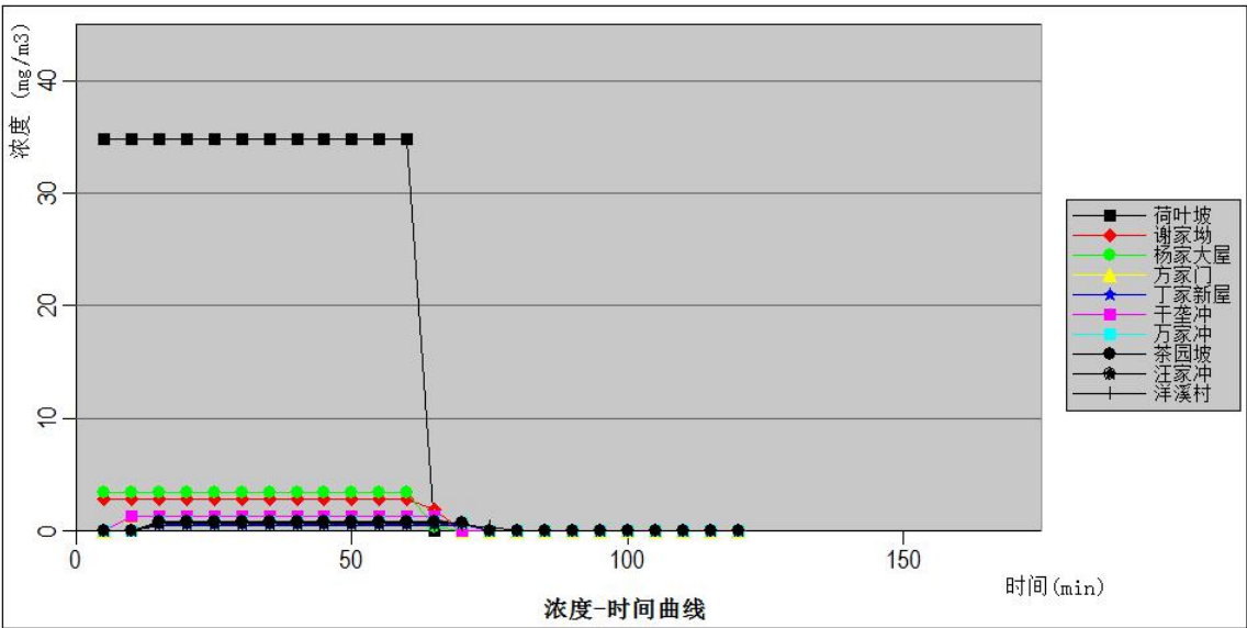
图 7.3.6-4a 主要关心点 CO 浓度随时间变化情况图（最不利气象条件）
