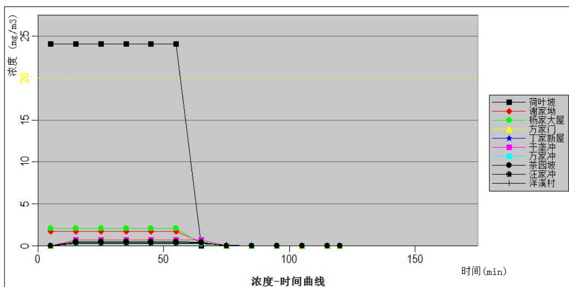
图 7.3.6-5b 主要关心点 HF 浓度随时间变化情况图（最常见气象条件）
