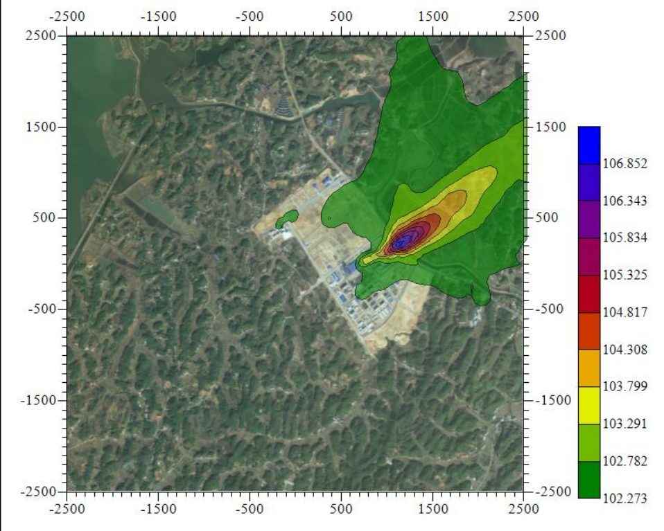
图 7.2.1.7-11a PM 10 日均值浓度叠加在建源及环境背景浓度预测结果分布图 (μg/m 3 )
