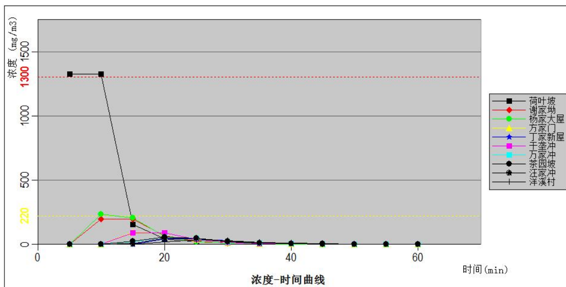
图 7.3.6-3a 主要关心点四氟乙烯浓度随时间变化情况图（最不利气象条件）
