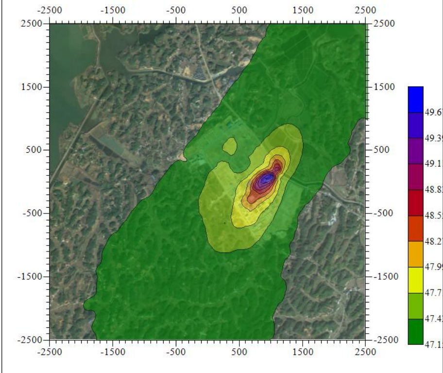
图 7.2.1.7-11b PM 10 年均值浓度叠加在建源及环境背景浓度预测结果分布图 (μg/m 3 )
