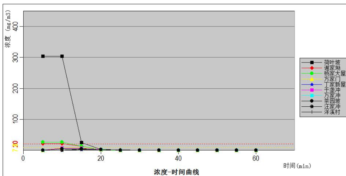
图 7.3.6-2b 主要关心点 F2 浓度随时间变化情况图（最常见气象条件）
