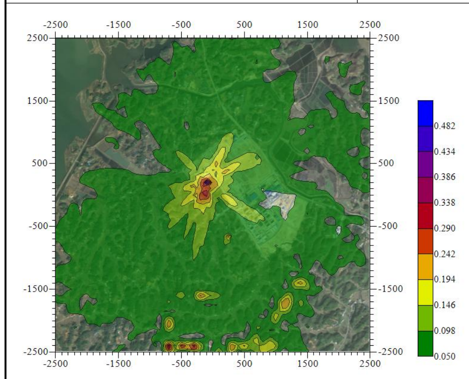
图 7.2.1.7-1a SO 2 小时平均浓度贡献值预测结果分布图 (μg/m 3 )
