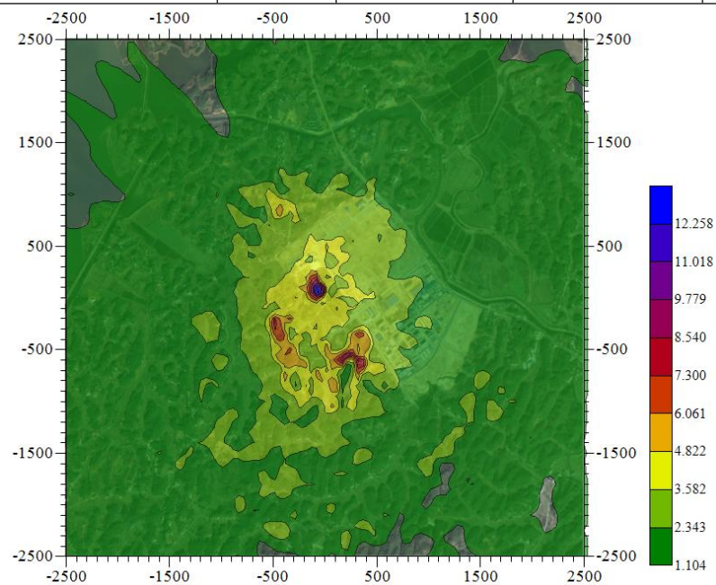
图 7.2.1.7-12a 氟化物小时值浓度叠加在建源及环境背景浓度预测结果分布图 ( \mu\text{g}/\text{m}^3 )
