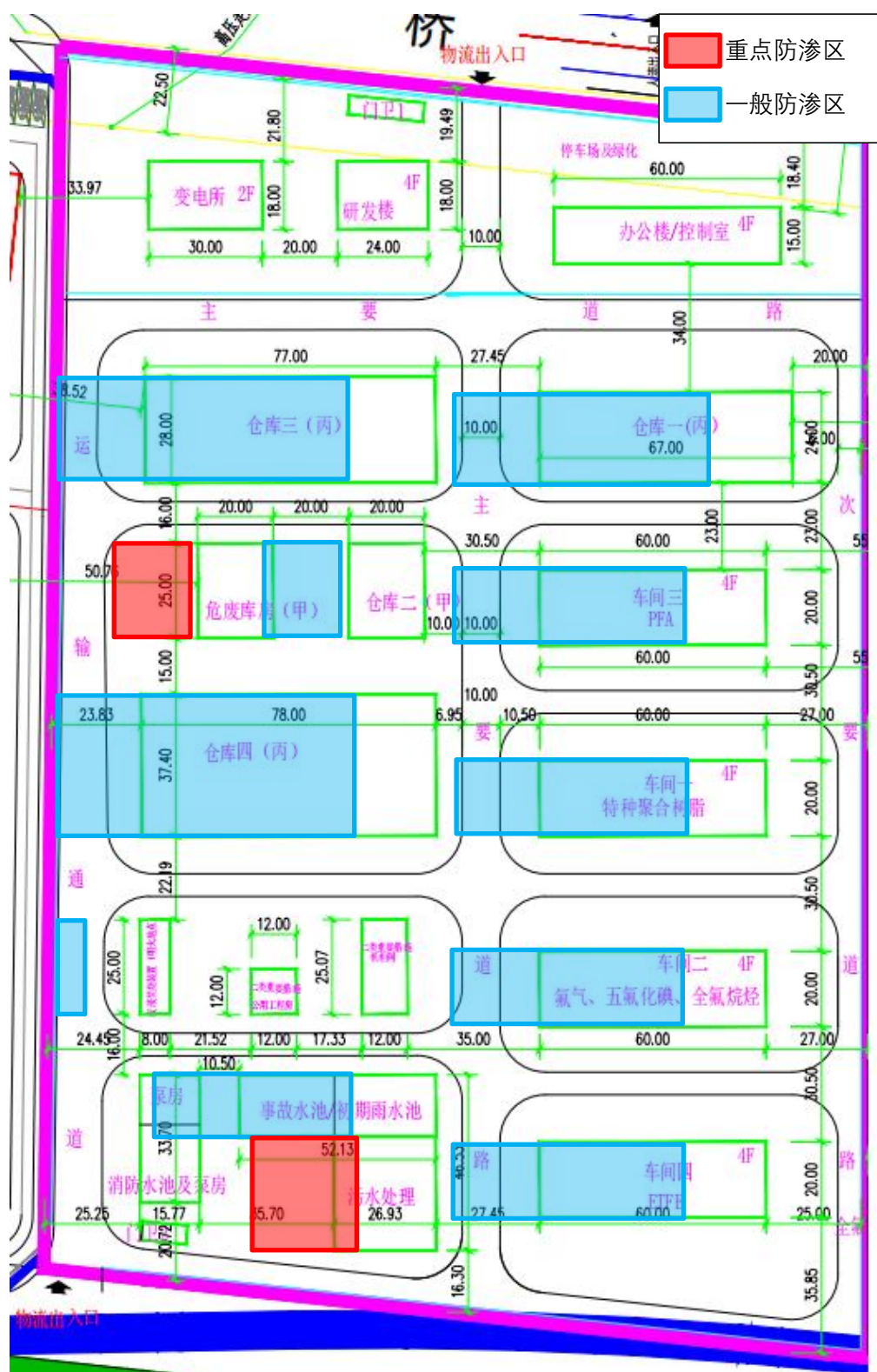
图 8.2-2 本项目地下水污染防渗分区示意图
