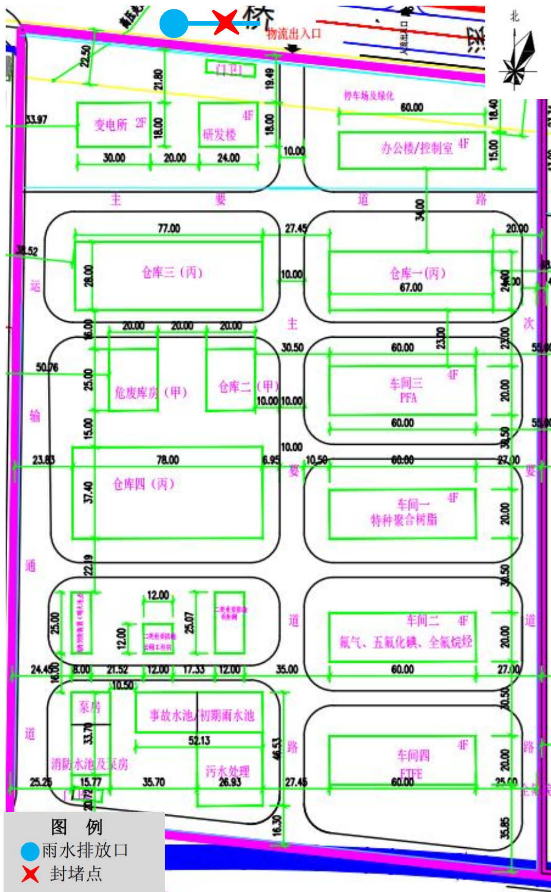
图 7.3.7-3 本项目防止事故废水进入外环境的控制、封堵系统图
