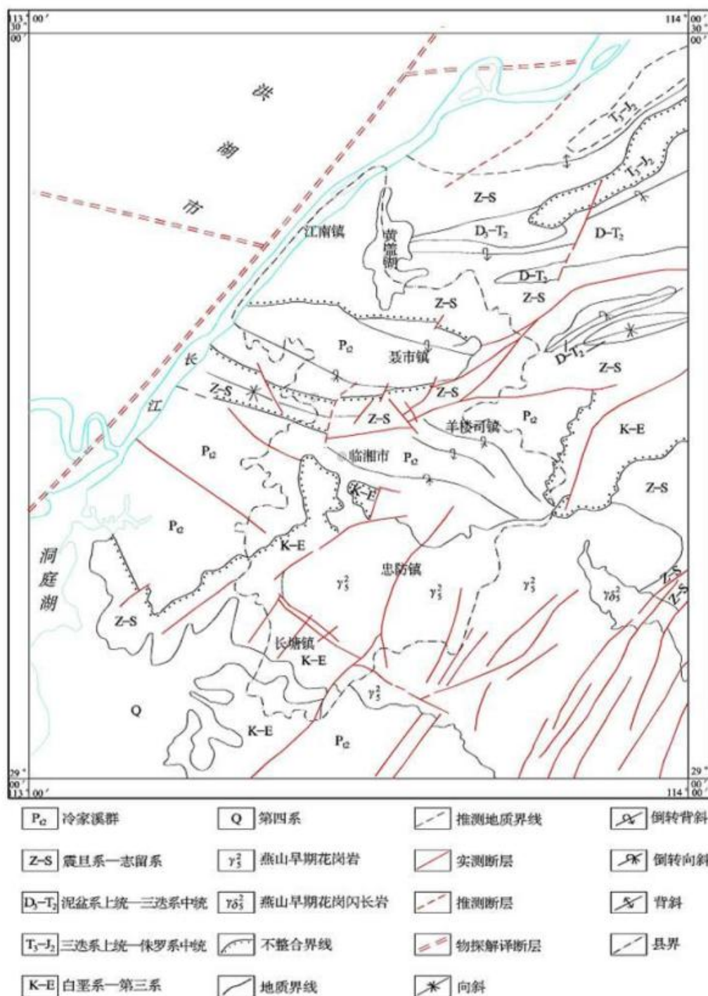
图 7.2.3-1 区域构造纲要图
