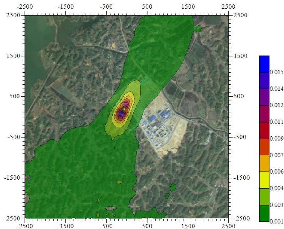
图 7.2.1.7-1c SO 2 年均浓度贡献值预测结果分布图 (μg/m 3 )
