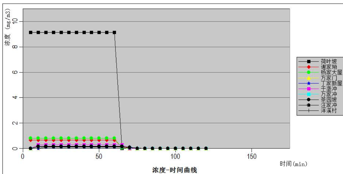
图 7.3.6-4b 主要关心点 CO 浓度随时间变化情况图（最常见气象条件）
