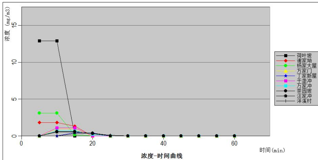
图 7.3.6-1b 主要关心点 HF 浓度随时间变化情况图（最常见气象条件）
