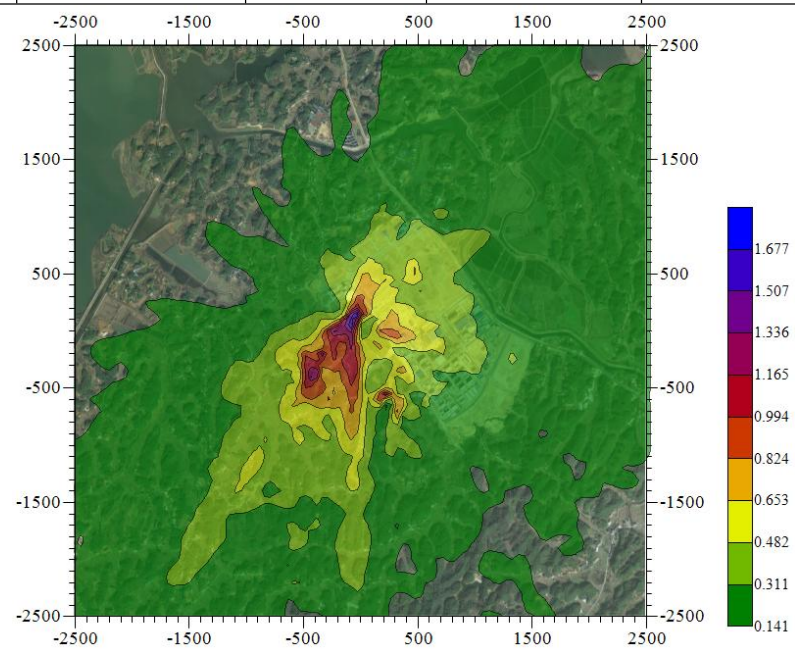
图 7.2.1.7-12b 氟化物日均值浓度叠加在建源及环境背景浓度预测结果分布图 ( \mu\text{g}/\text{m}^3 )
