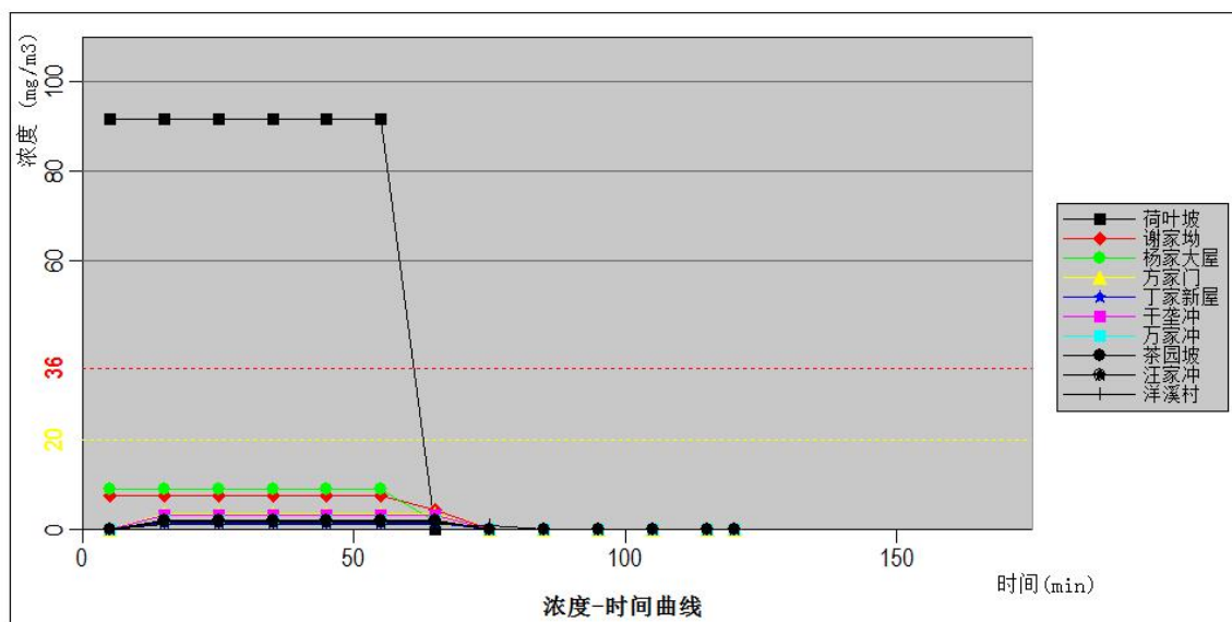
图 7.3.6-5a 主要关心点 HF 浓度随时间变化情况图（最不利气象条件）
