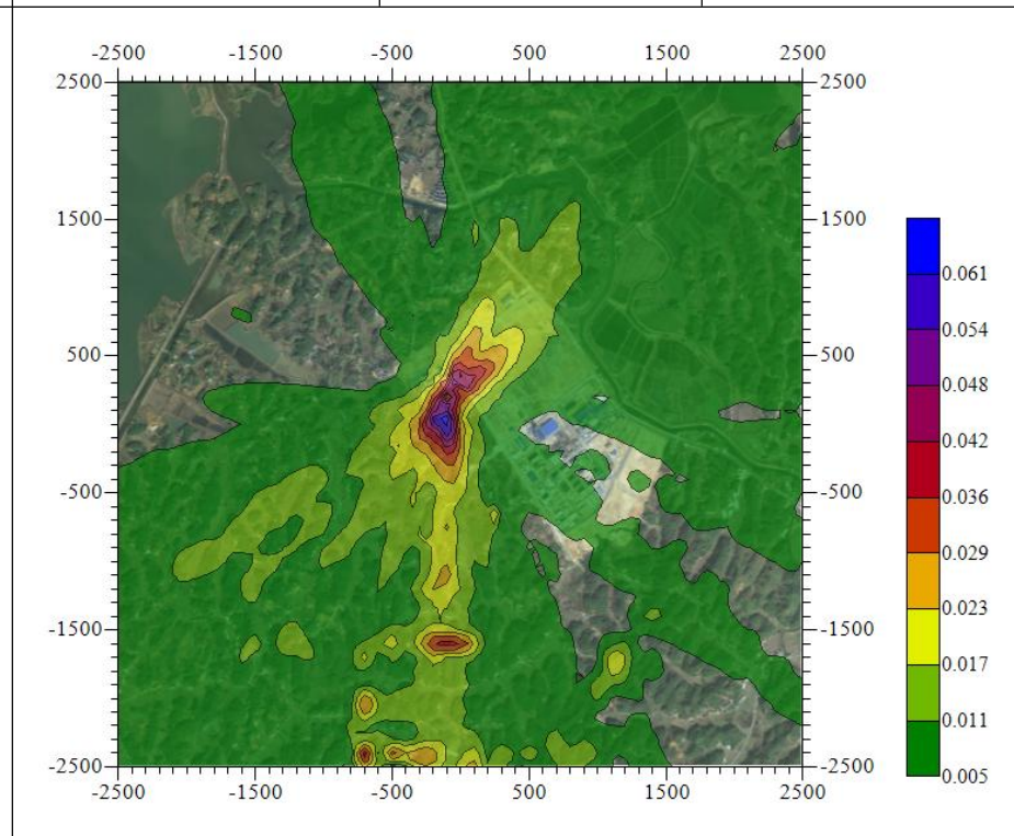
图 7.2.1.7-1b SO 2 日均浓度贡献值预测结果分布图 (μg/m 3 )
