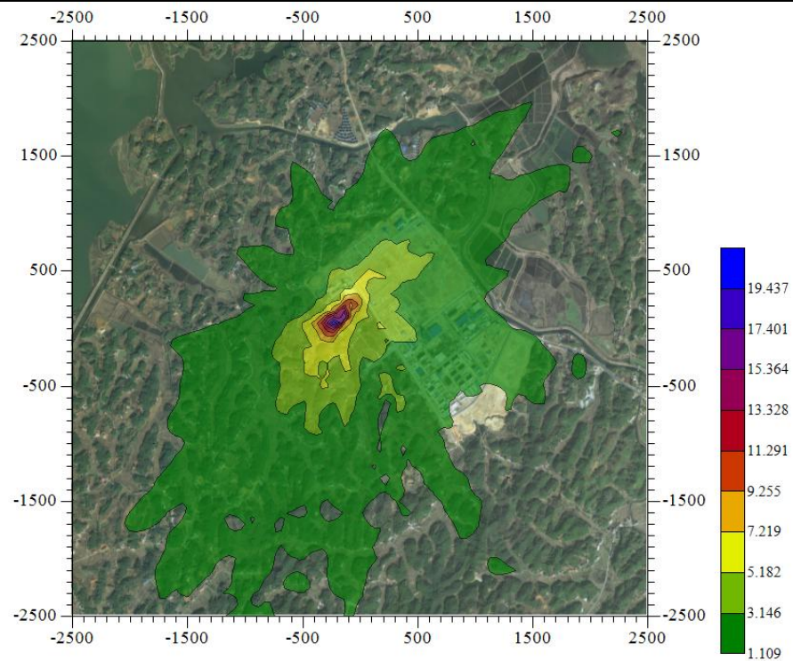
图 7.2.1.7-8 TVOC8 小时浓度贡献值预测结果分布图 ( \mu\text{g}/\text{m}^3 )
