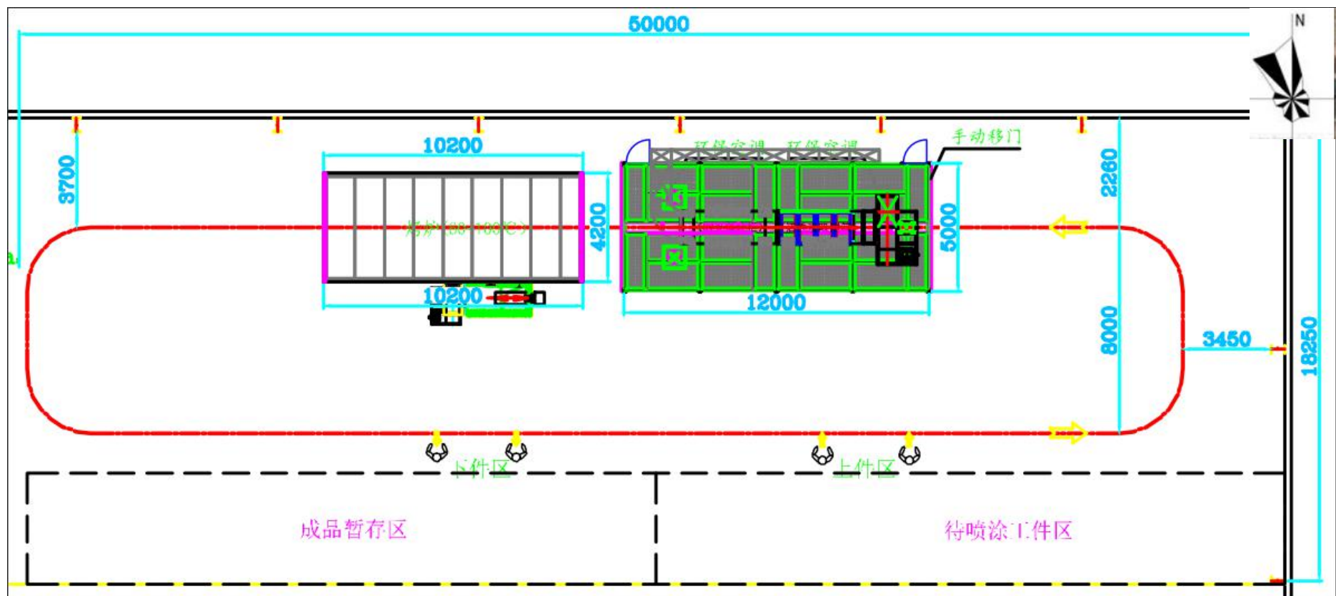
附图三 喷漆、烘干上下工件示意图
