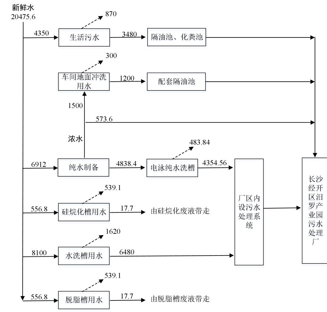
图 3.4-1 水平衡图 单位: m³/a
