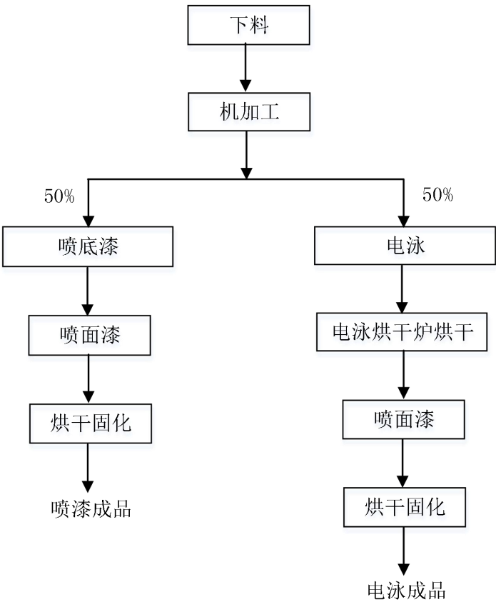
图 3.3-1 总体工艺流程示意图
