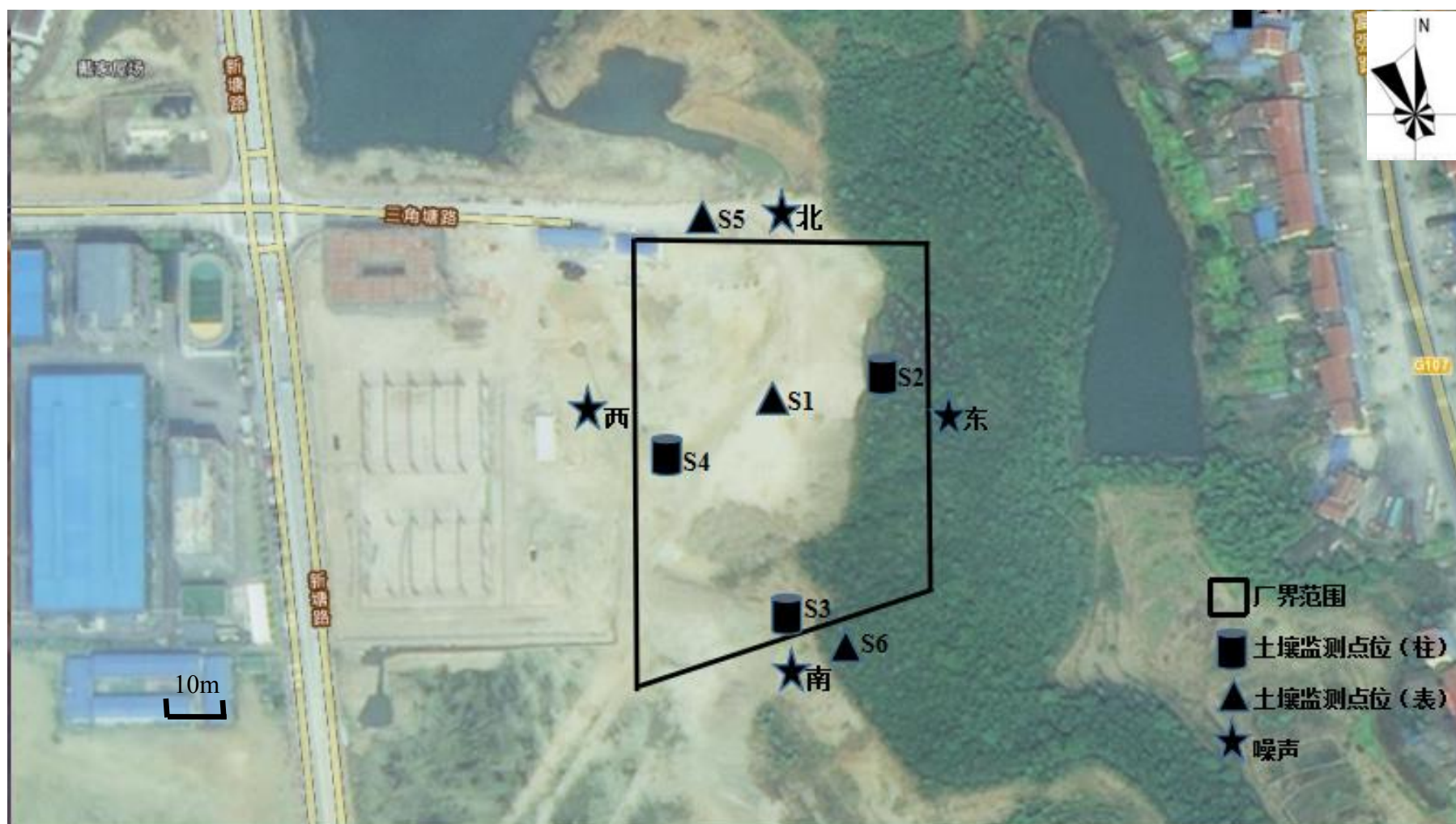
附图四 土壤、噪声监测布点图
