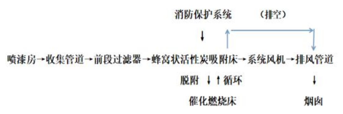
图 6.2-1 废气处理示意图
