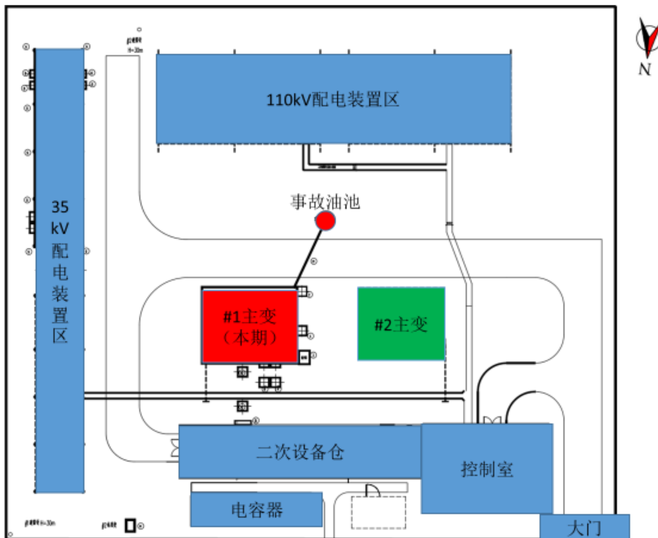
附图二 操军 110kV 变电站总平面布置图
