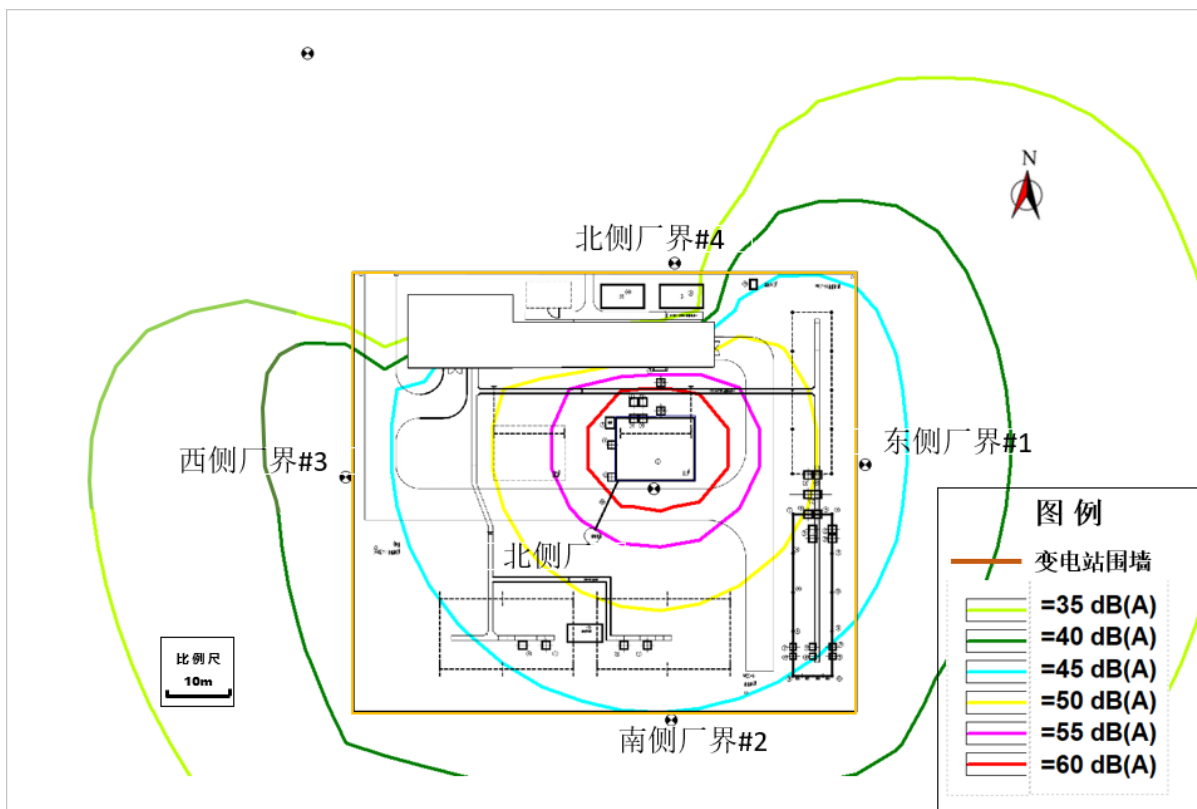
图 8 操军 110kV 变电站本期规模噪声预测等值线图
