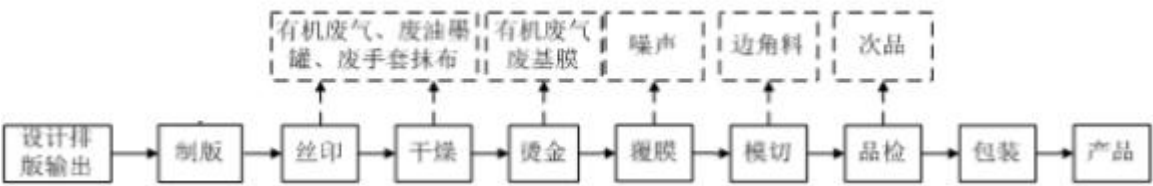
图 5-1 丝印生产工艺流程图
