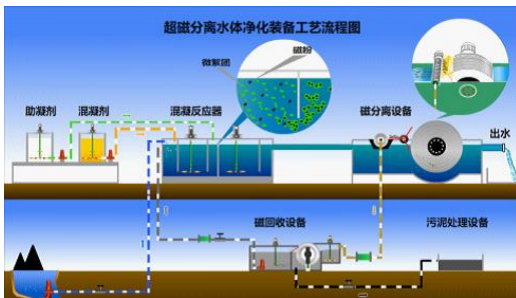
图 3.4-2 超磁分离水体净化工艺流程图
