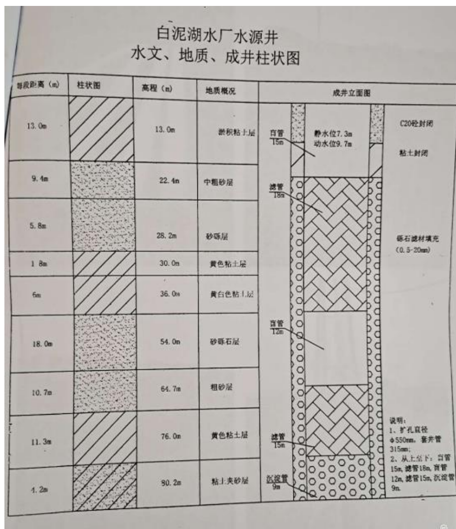
图 6.1-2 白泥湖水厂水源井水文、地质、成井柱状图
