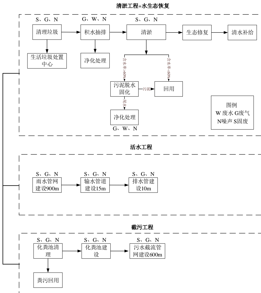
图 4.2-1 黑臭水体污染整治流程图
