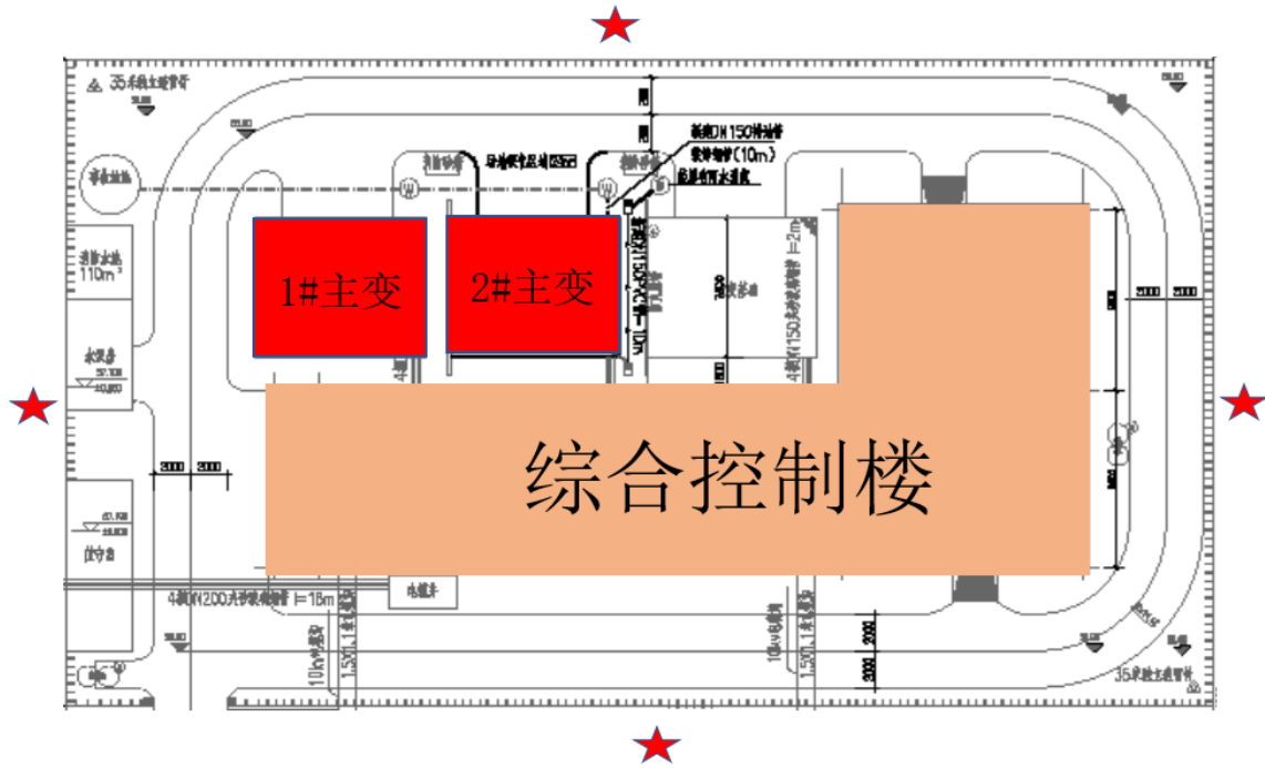
图 4 富民 110kV 变电站平面布置及监测点位示意图
