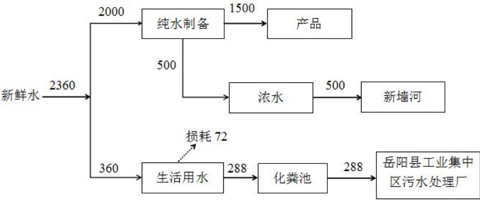
图 3.3-1 项目水平衡图 单位：m³/a
