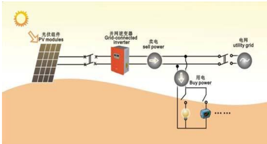
图5-4 光伏发电系统原理结构图
