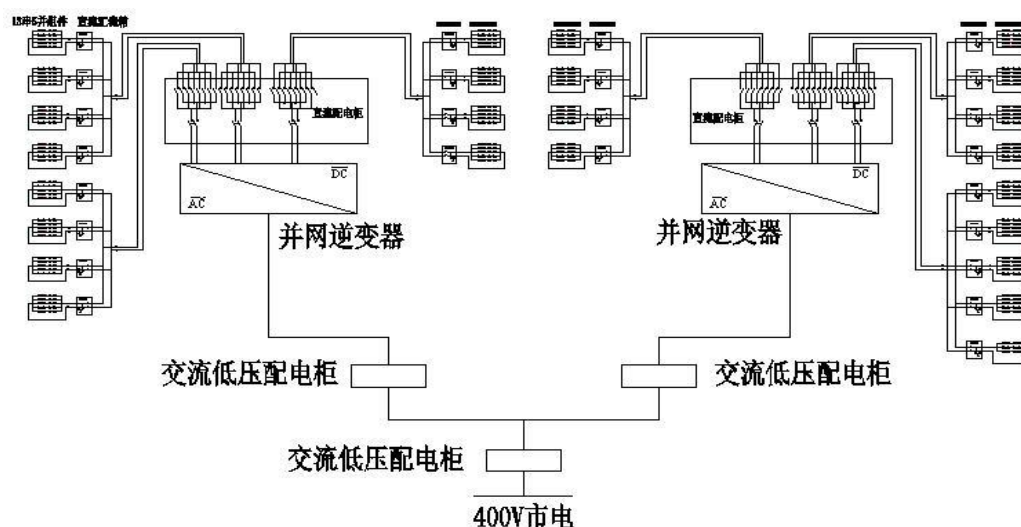
光伏系统并网接线框图
