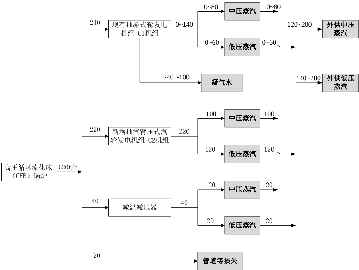
图3 实施本次改造（改造后）后蒸汽平衡图（单位 t/h）
