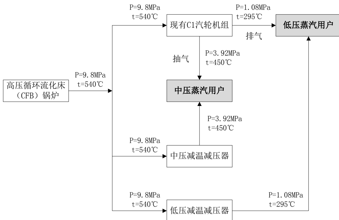
图1 不实施本次改造（改造前）供热方案示意图
