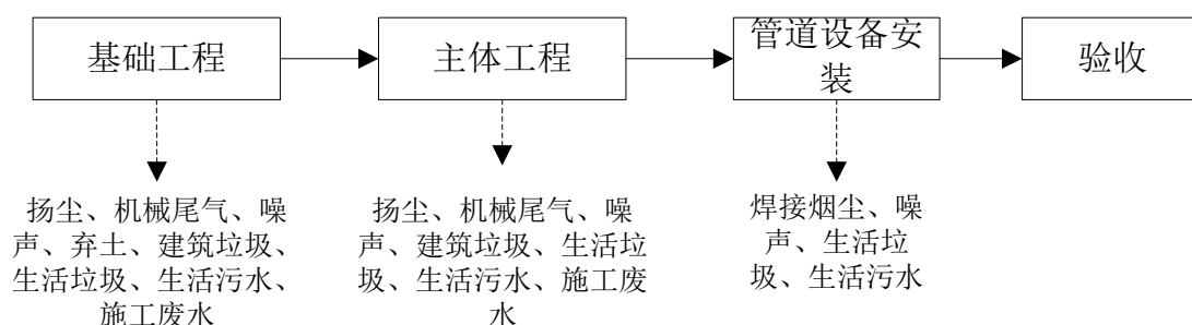
图4 施工期工艺流程及产污节点图
