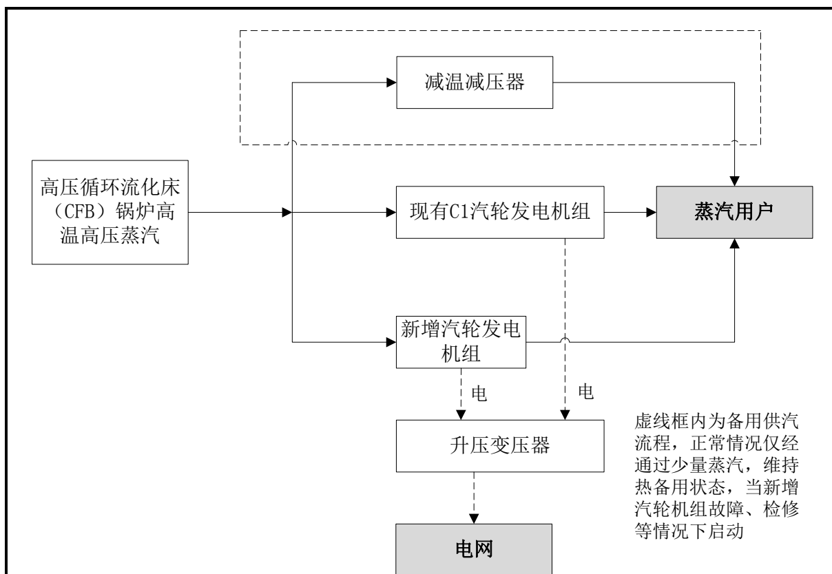
图5 项目运营期工艺流程图
