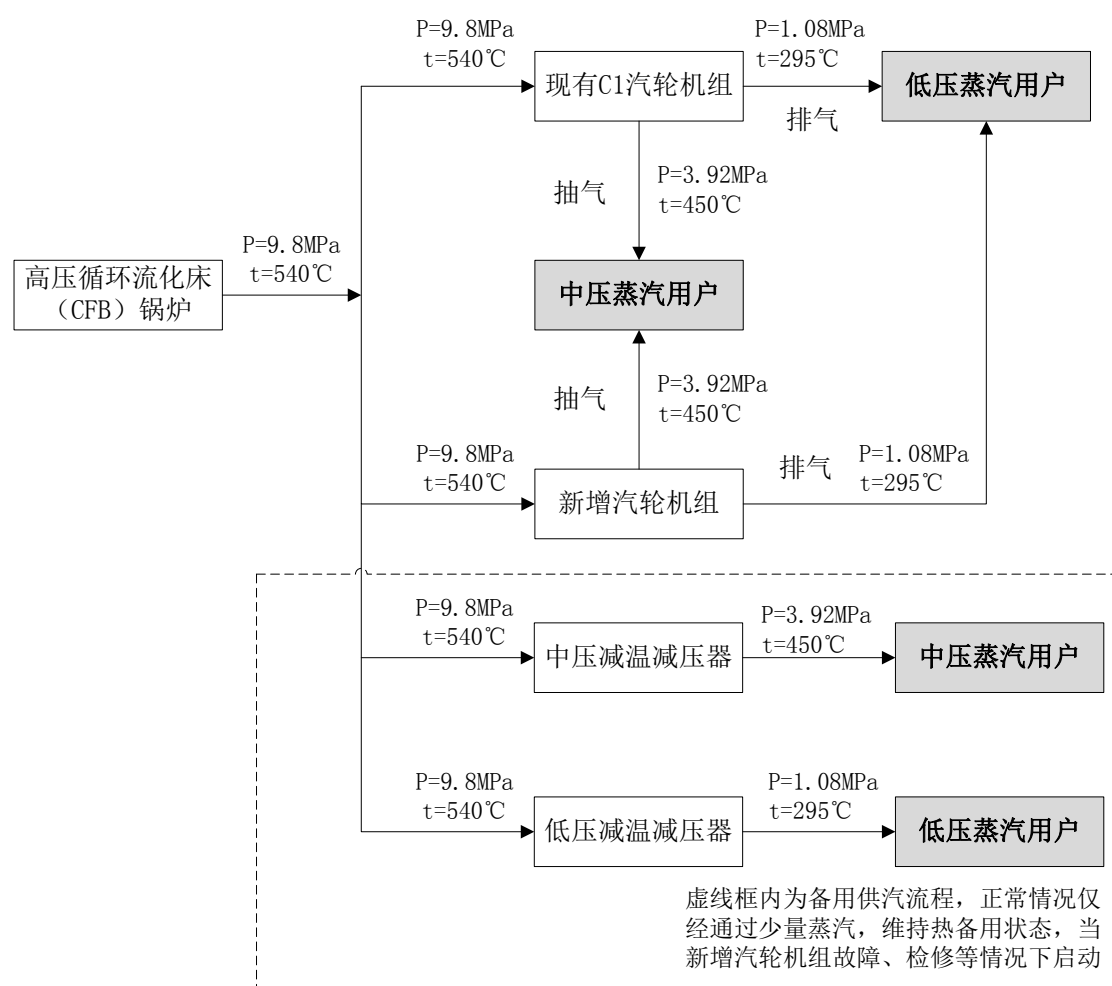
图2 实施本次改造（改造后）供热方案示意图
