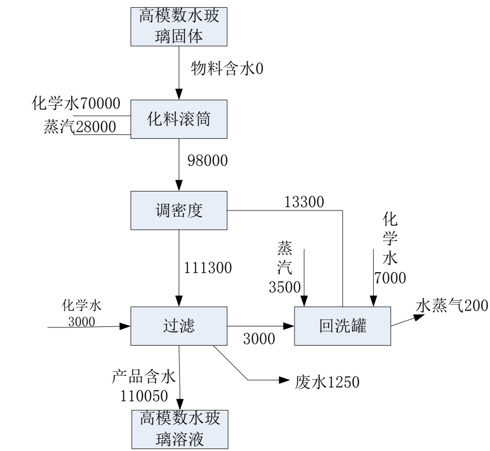
图 3-3 水玻璃产品生产水平衡图（单位：t/a）
