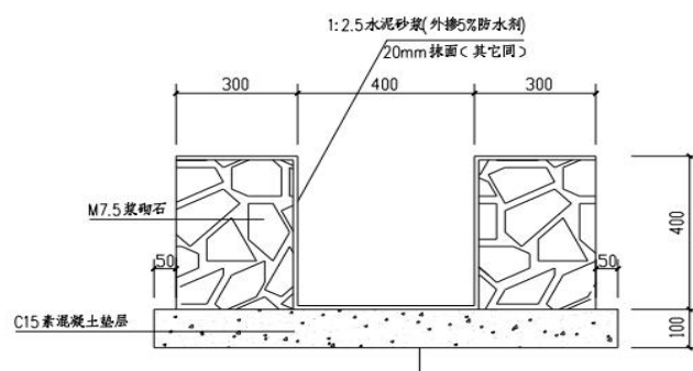
图 2.6-8 坡面排水沟示意图
