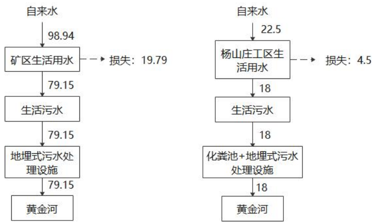
图 2.1-12 生活污水水平衡图 (m³/d)
