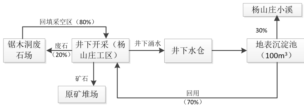
图 2.1-4 杨山庄工区采矿工艺流程图（现有）
